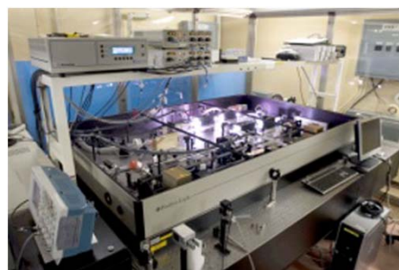
EUV光源プラズマ装置
