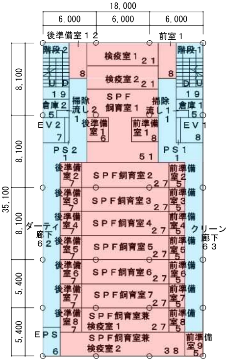
3 階平面図 6 3 2 m 2
