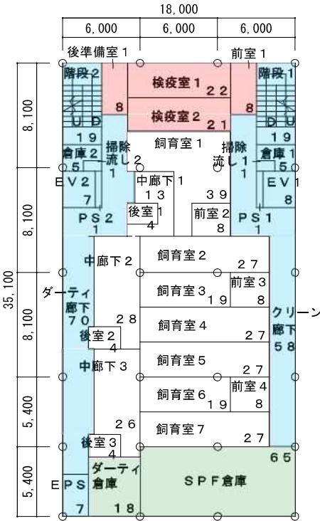
2階平面図 632㎡
