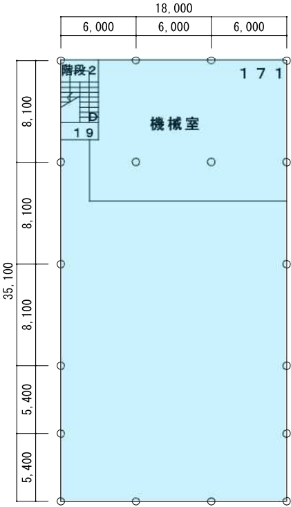
4 階平面図 1 9 0 m 2
