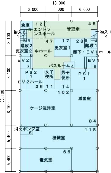
1階平面図 632㎡
