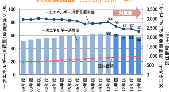
主要3キャンパス（吹田・豊中・箕面）のエネルギー消費量推移
