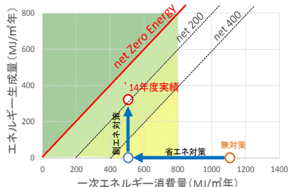
登録有形文化財でのnZEB化を目指した改修
