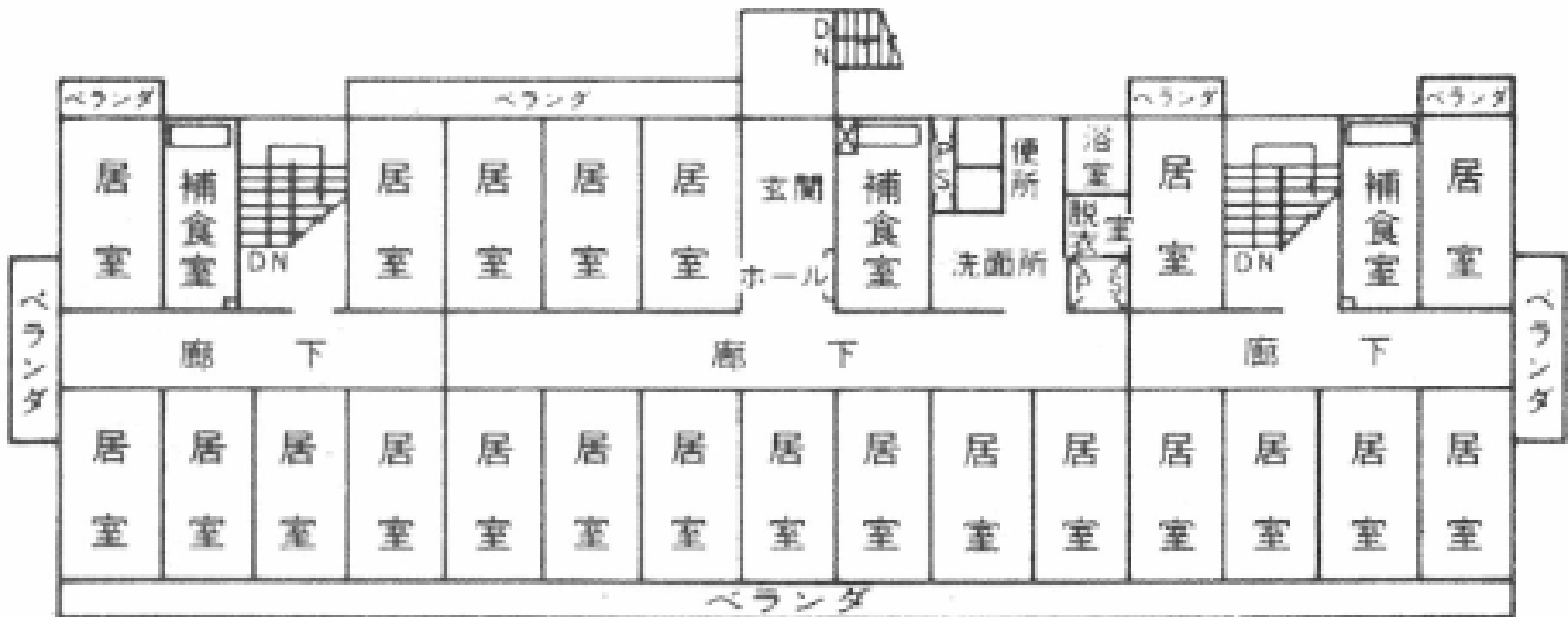
2階平面図
