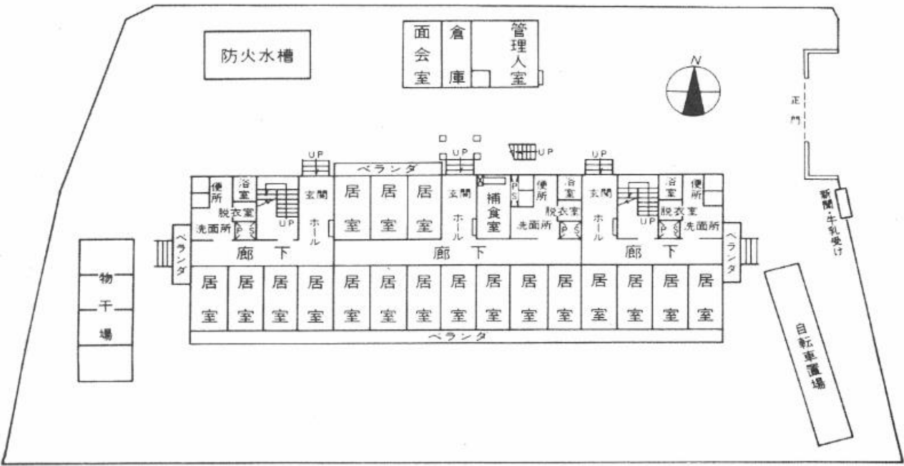
1階平面図
