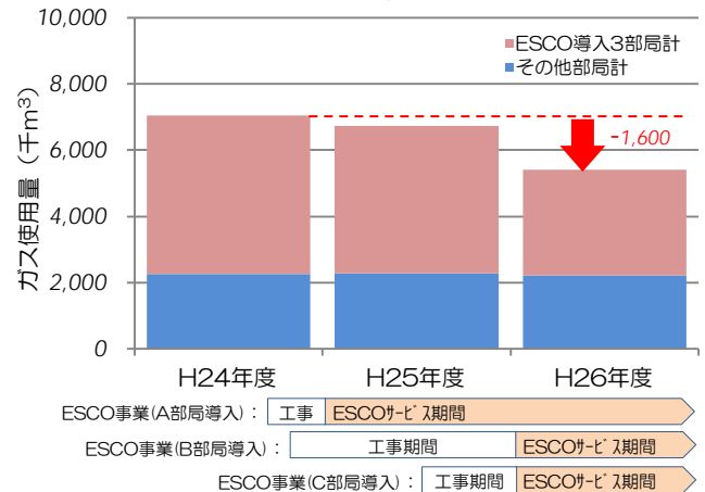
ガス使用量の推移(吹田キャンパス)
